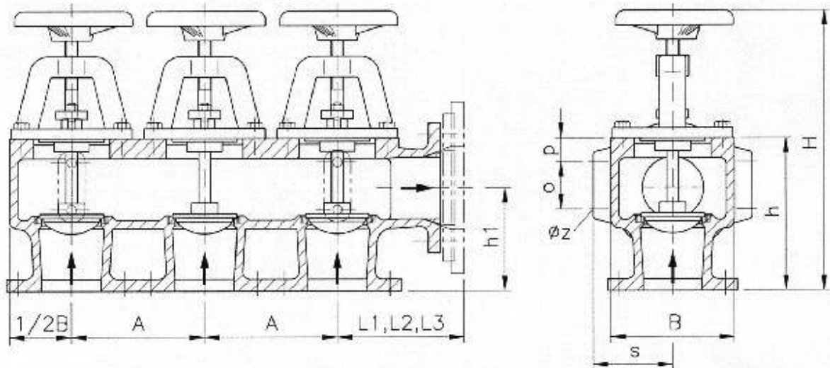
Type 019615 Sauge-Ventilkasten (Beispielabbildung) Type 019615 suction valve chest (example)
